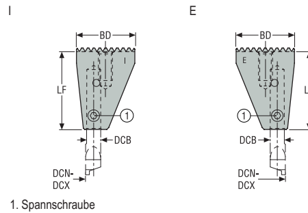
1. Spannschraube
