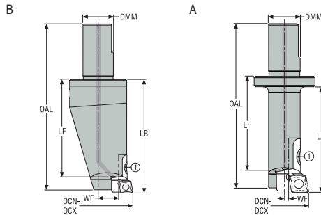
1 = Spannschraube
